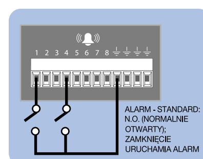
Ryc. 5. Kocówki alarmowe
